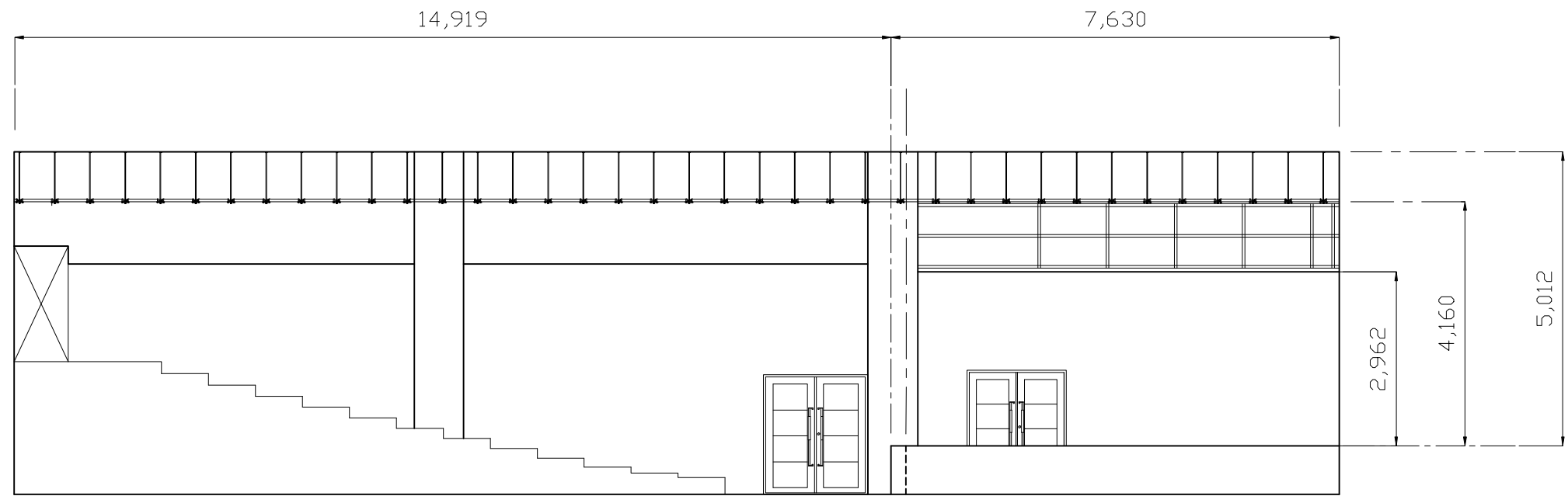
소극장 블루 우측면도
